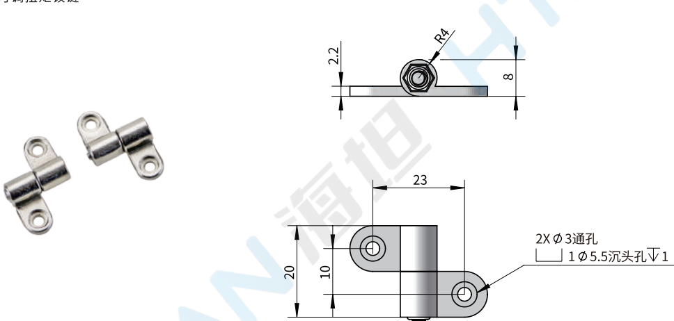
■ 可调扭矩铰链
