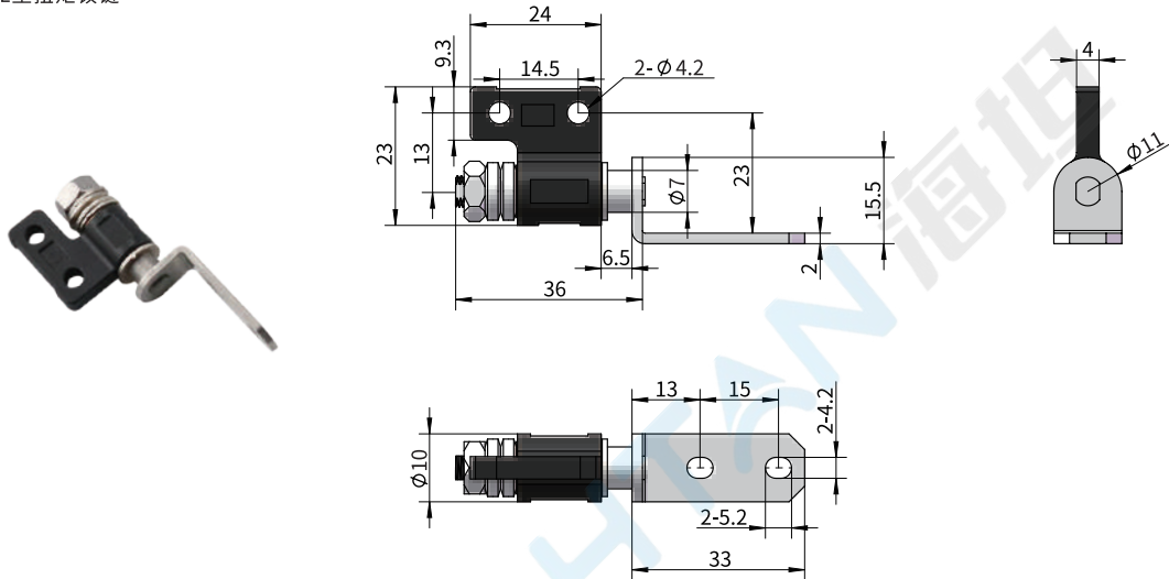
■ L型扭矩铰链
