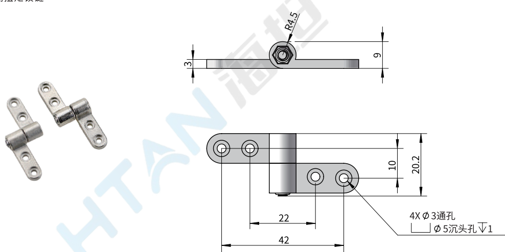
■ 可调扭矩铰链
