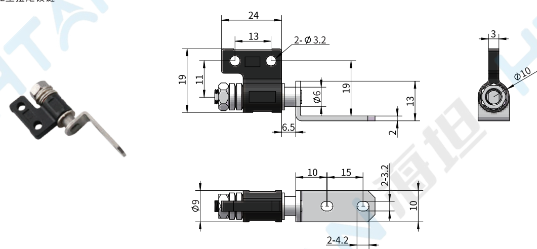
■ L型扭矩铰链
