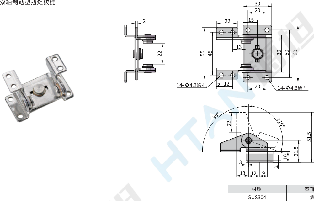
■ 双轴制动型扭矩铰链
