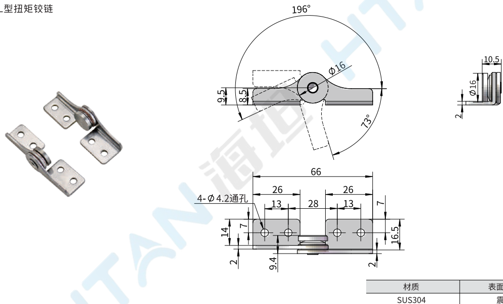
■ L型扭矩铰链
