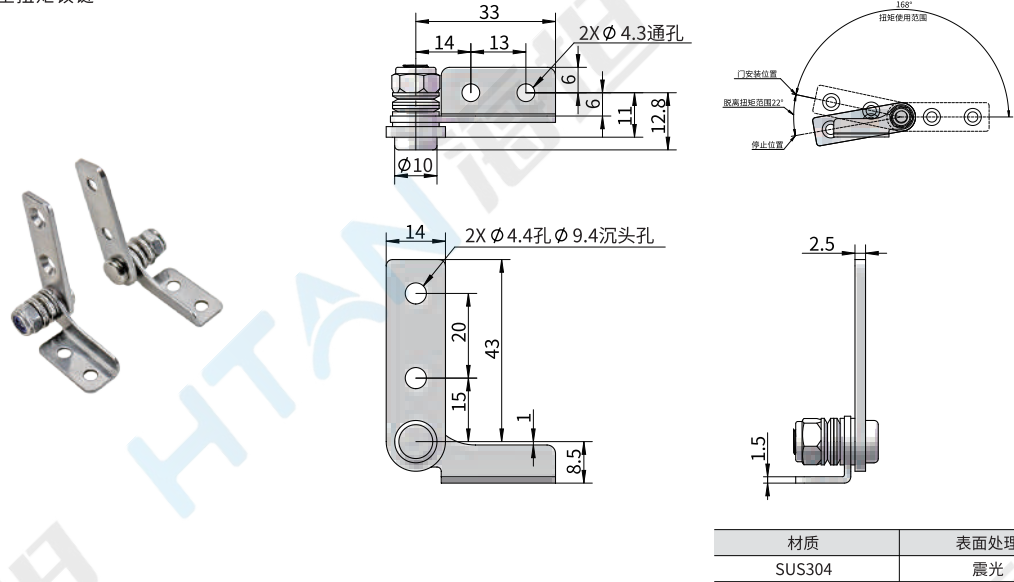
■ L型扭矩铰链
